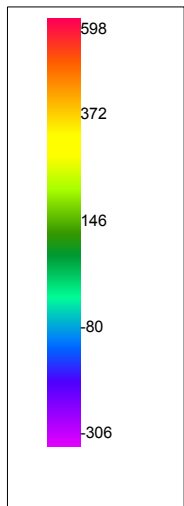
Regional gravity survey data.
