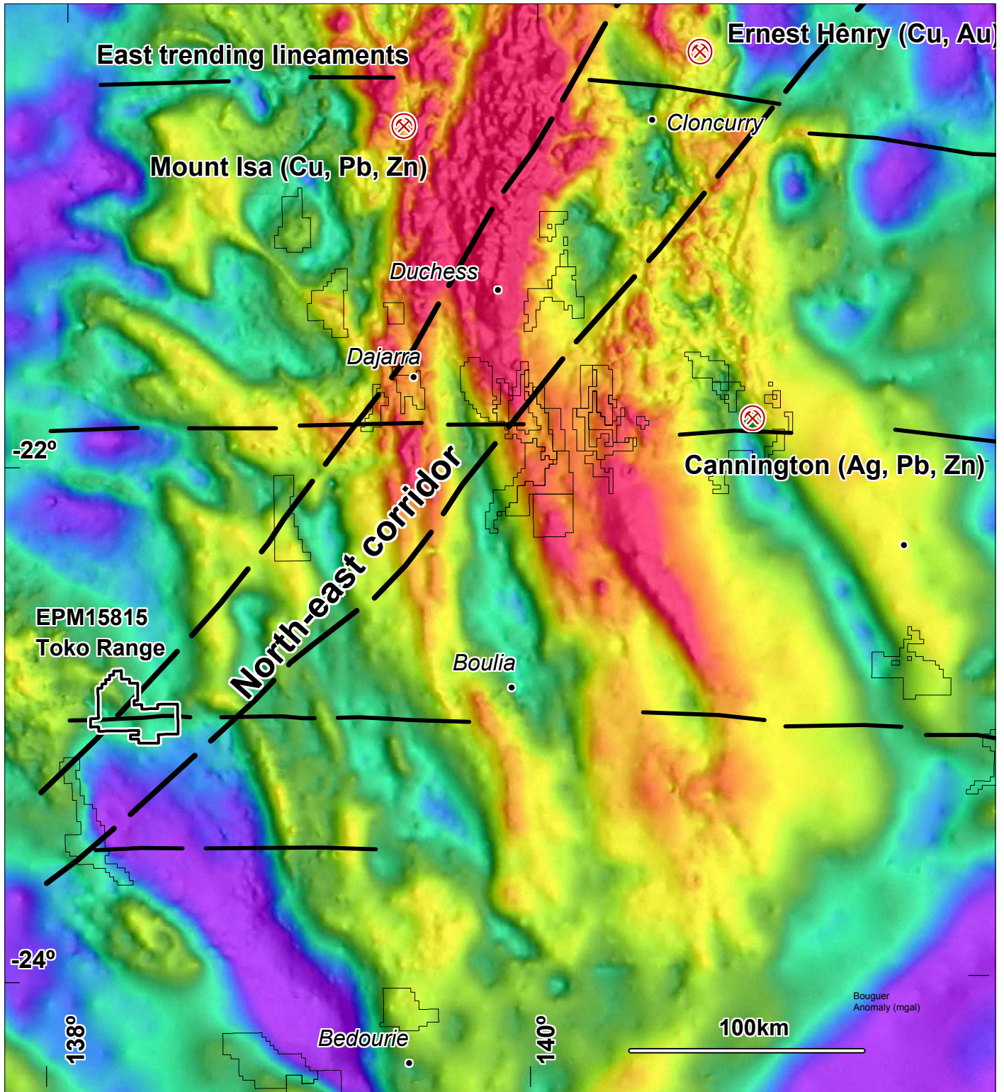
Regional gravity survey data.
